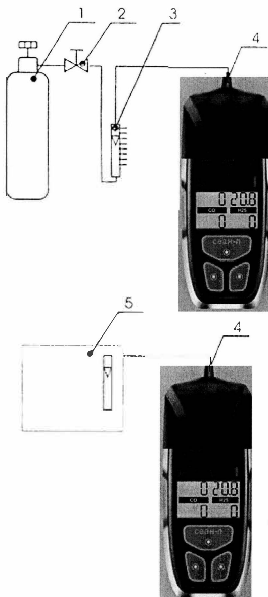
Рис. 1. - Схема соединения газоанализатора с источником ПГС 1 - баллон с ПГС, 2 – вентиль, 3 – ротаметр, 4 – градуировочная насадка, 5 - генератор ПГС
