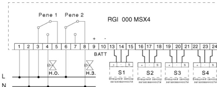
Рис.2 Схема подключения
