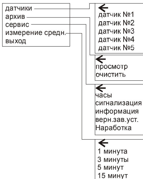
Рисунок 2.3 Меню газоанализатора
