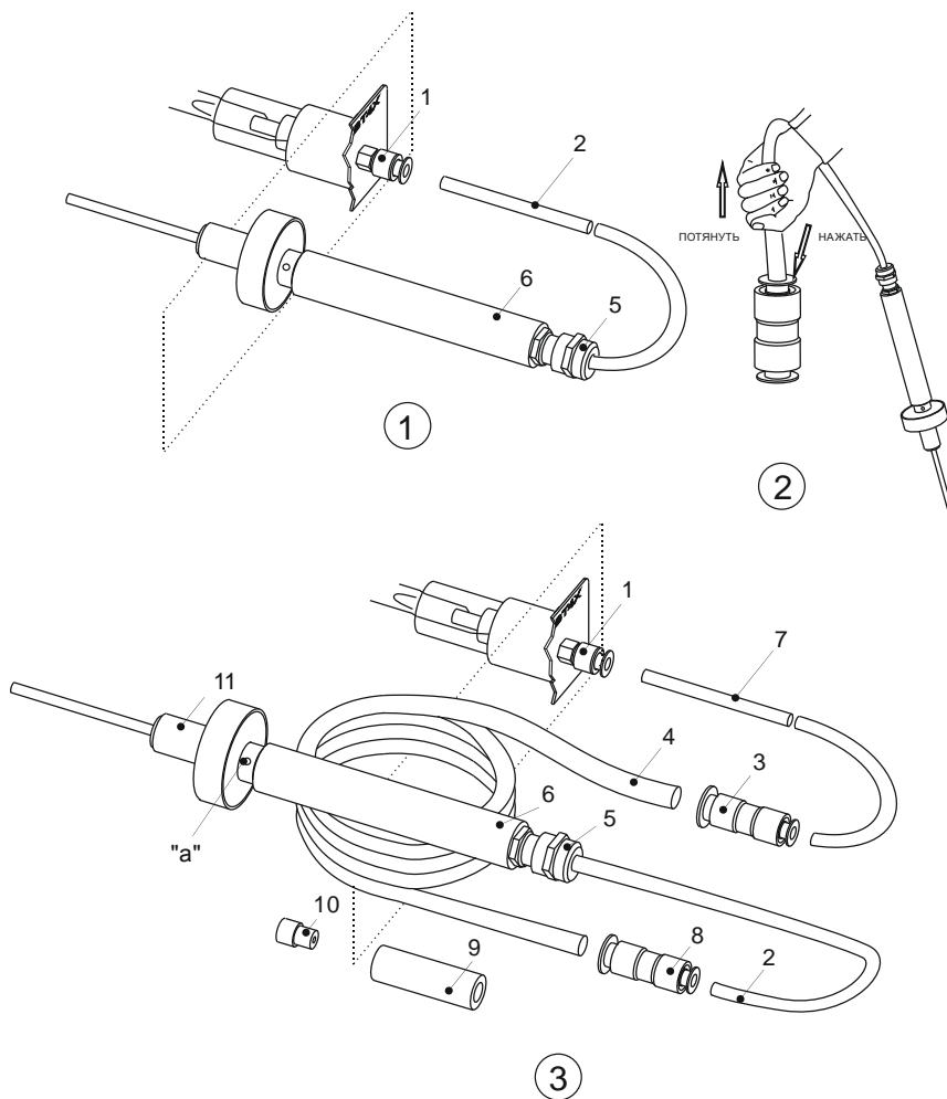
Рис. 4. Схема соединения элементов пробоотборника с газоанализатором (1) и элементов удлинителя с газоанализатором (2)
