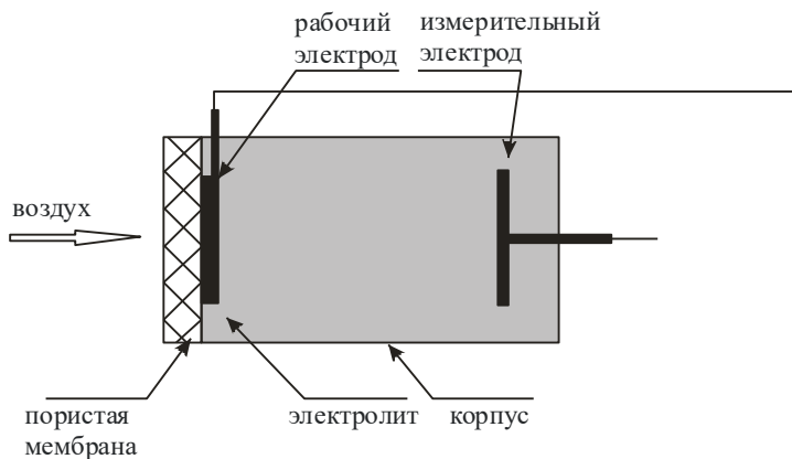
Рис. 1. Электрохимический детектор
