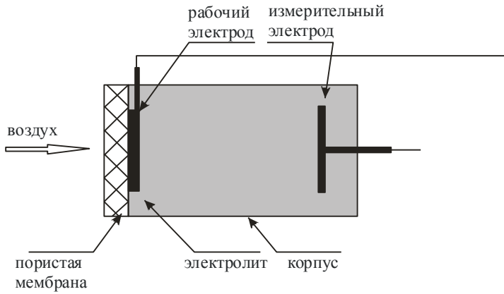
Рис. 1. Электрохимический детектор
