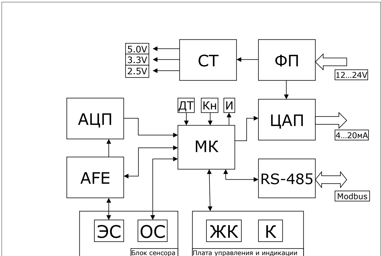
Рис. 3 Структурная схема газоанализатора
