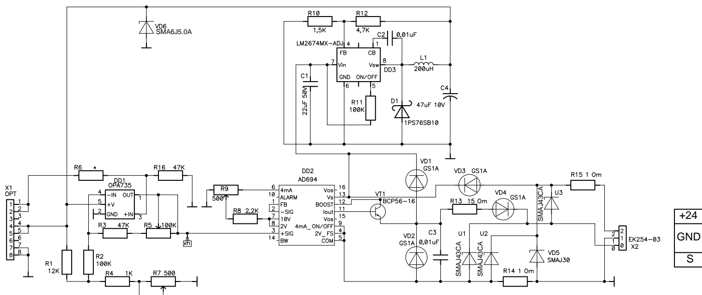
Схема электрическая датчиков с оптическим сенсором (Бином-Д, Верба-Д, Марш-Д и Дукат-Д)
