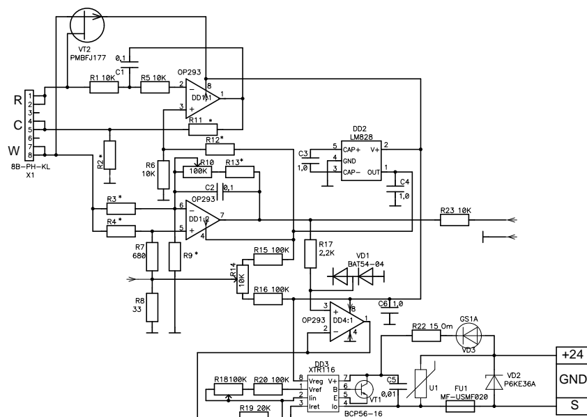
Рис 1 принципиальная схема электронной платы ЕС-А8М для электрохимических сенсоров, прибор ФГИМ 413415.001-400-004-001.
