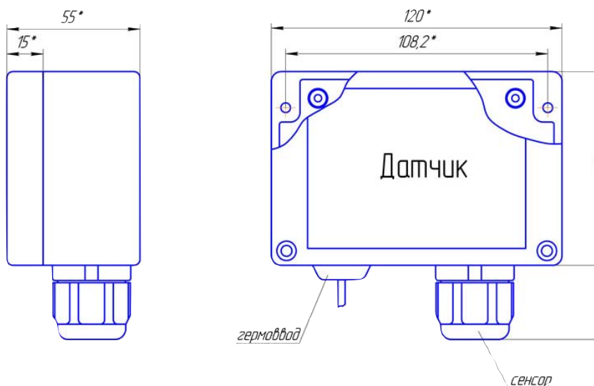
Рис. 2. Габариты датчика в пластиковом корпусе со встроенным сенсором (ФГИМ 413415.001-400-004-001)
