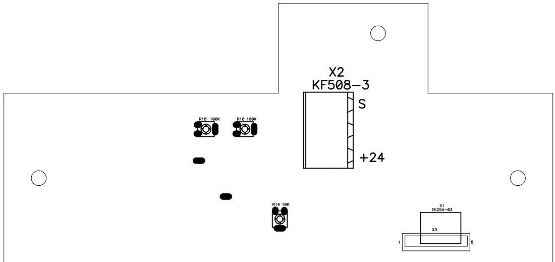
рис.1а. Расположение элементов на плате ЕС-А8М с обратной стороны, прибор ФГИМ 413415.001-400-004-001.
