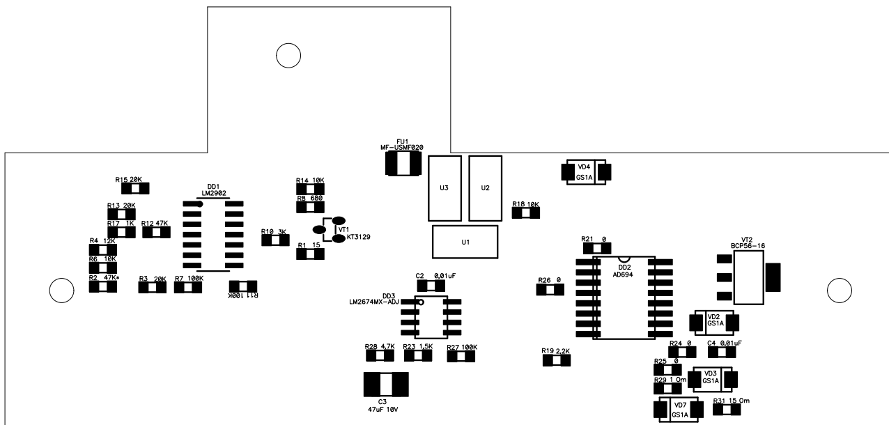
Рис.26. Расположение элементов на плате ТК-А8М с лицевой стороны, прибор ФГИМ 413415.001-400-004-001.
