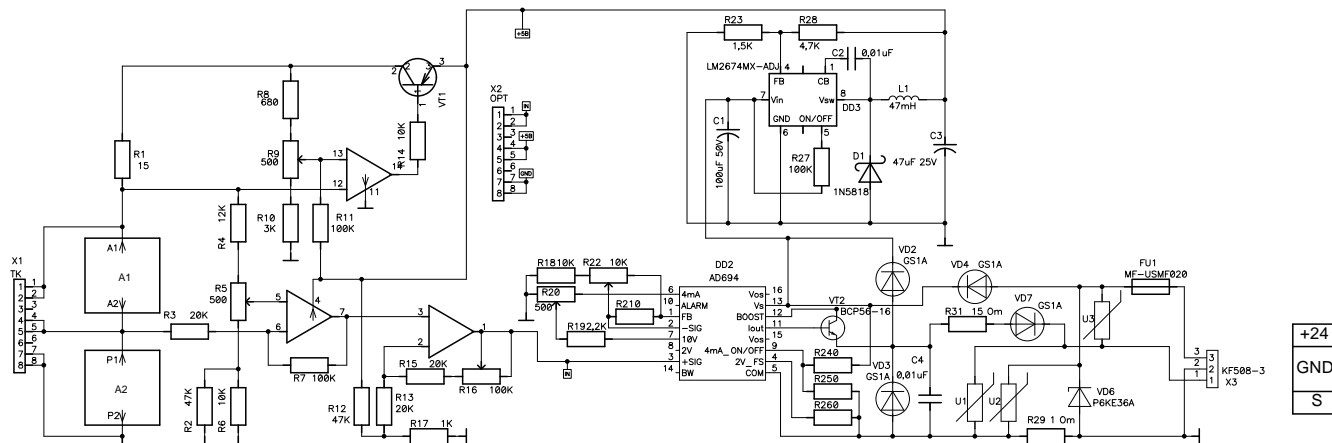
Рис 2 принципиальная схема электронной платы ТК- А8М для электрохимических сенсоров, прибор ФГИМ 413415.001-400-004-001.
