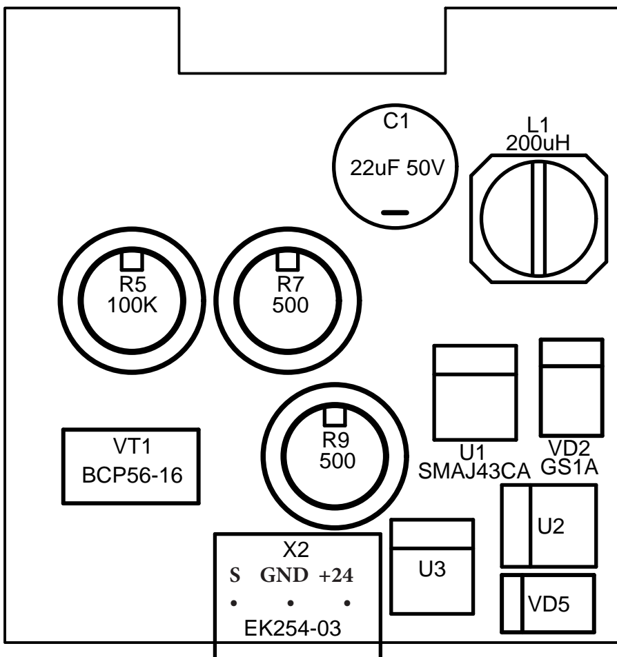
Монтажная схема платы OP-DU v 1.2. Вид снизу
