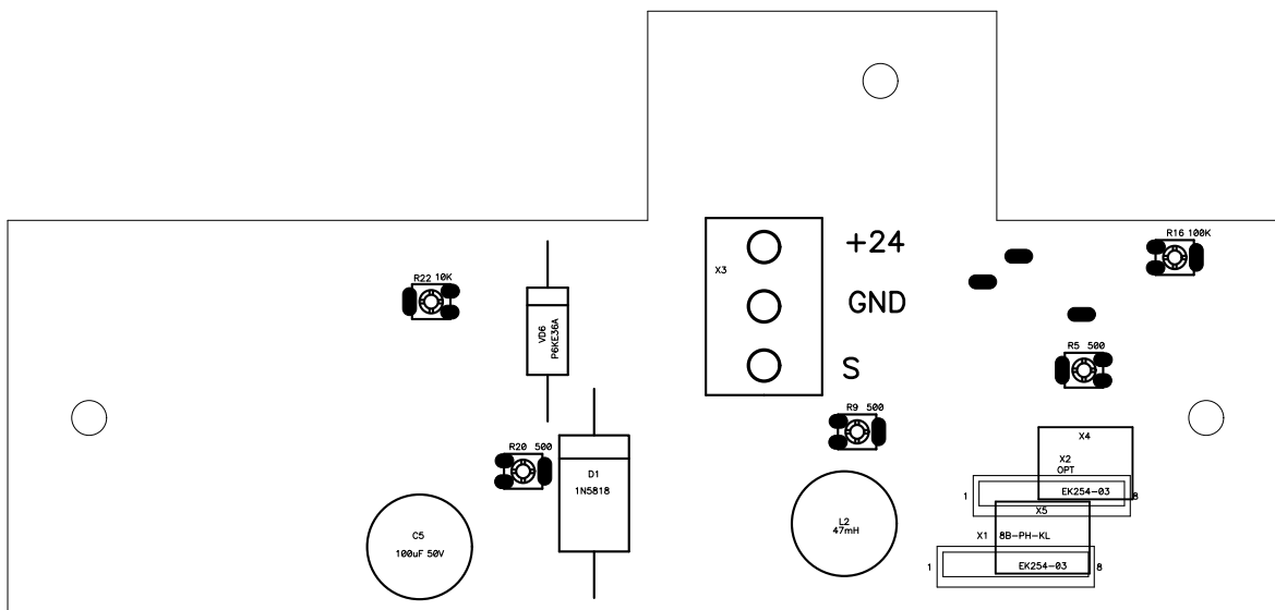
рис.2а. Расположение элементов на плате ТК-А8М с обратной стороны, прибор ФГИМ 413415.001-400-004-001.
