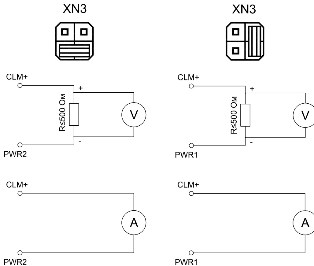
Рисунок Б.2 – Установка перемычки XN3 при подключении по трехпроводной линии: 2 провода питания и один провод CLM+ (активная токовая петля).
