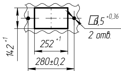
Разметка щита для установки газоанализатора
