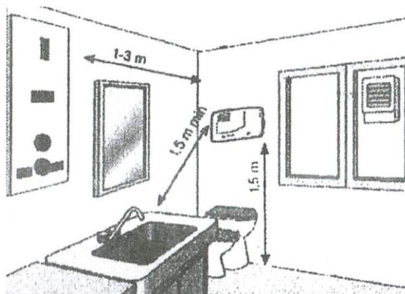
Рисунок 1А - Схема места установки сигнализатора
