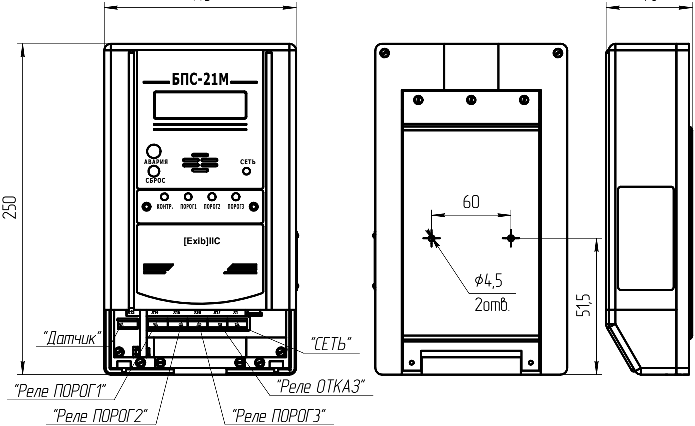
а) блок БПС-21М-1ВБ
