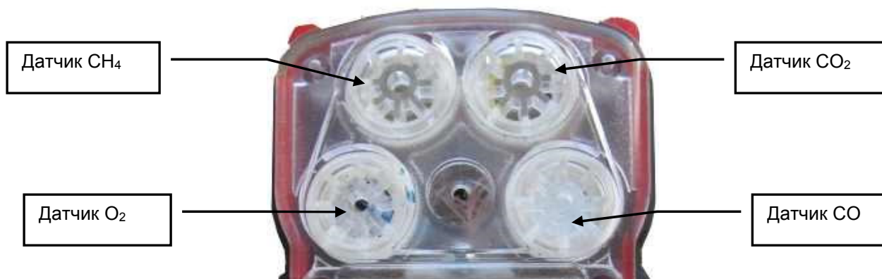
Рис. 3. Схема расположения газопроницаемых входов датчиков
