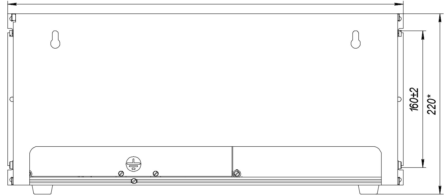
Вид сзади 480*
