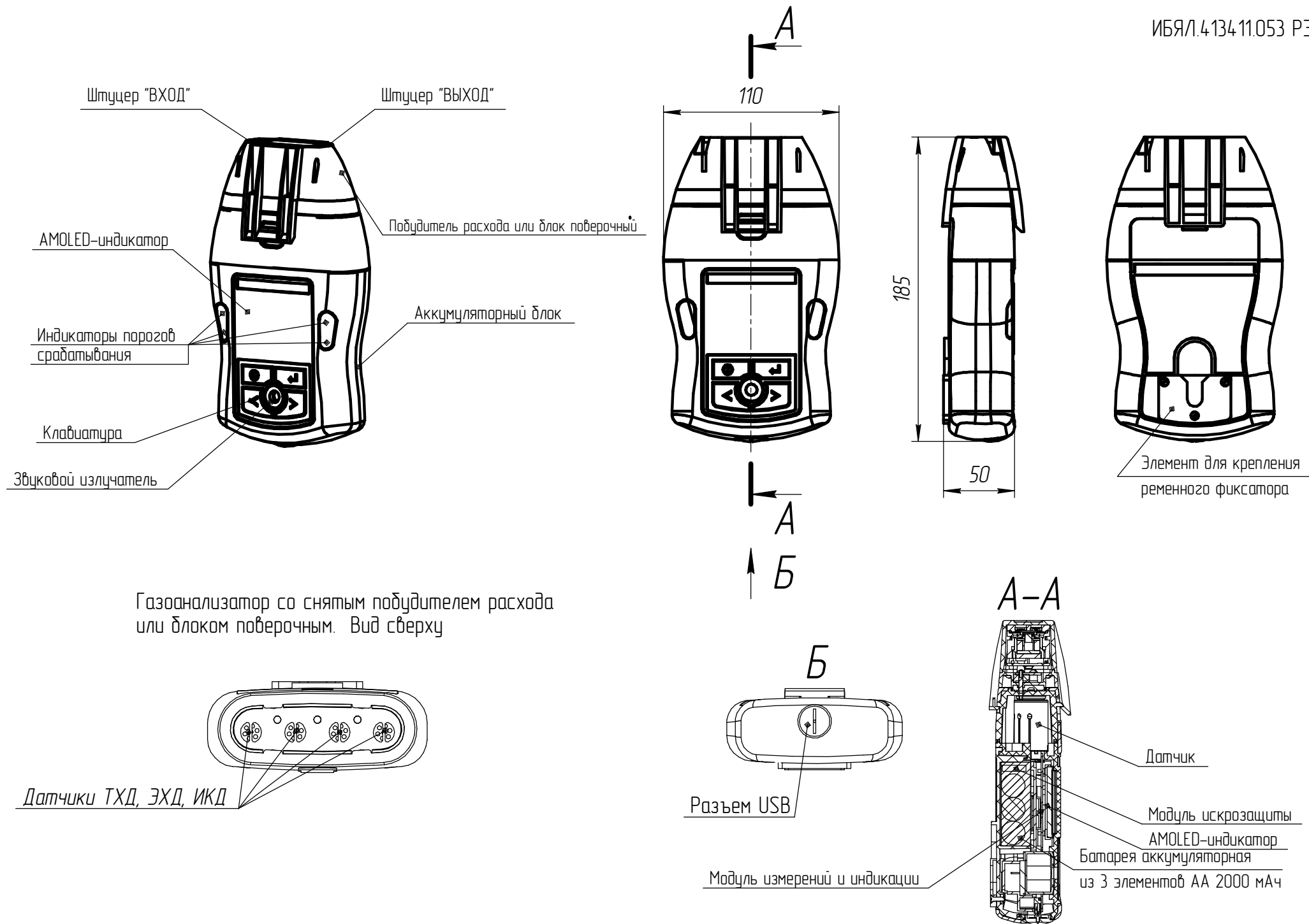
Рисунок 1.1 – Газоанализаторы АНКАТ-7664Микро ... -16. Внешний вид
