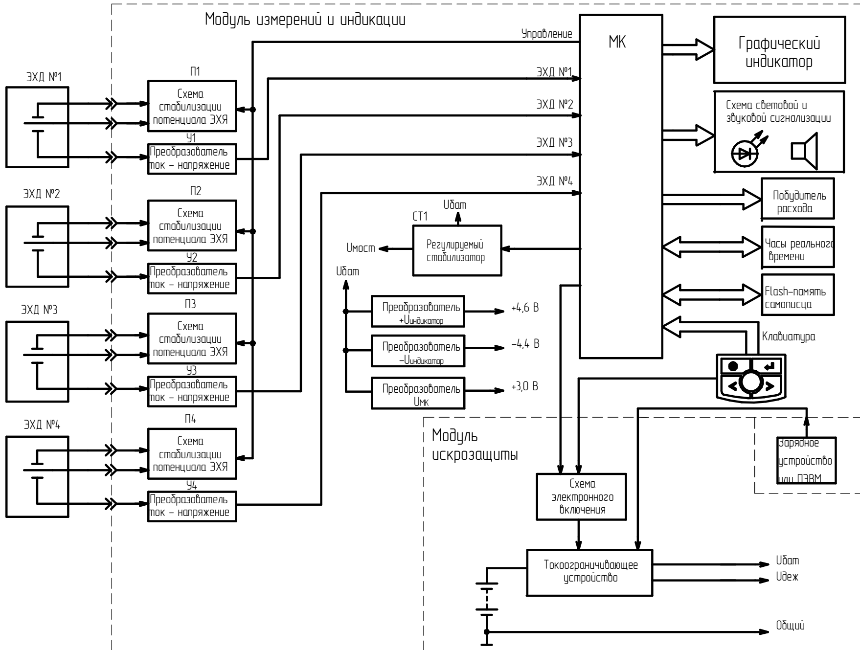
Рисунок 1.3 – Газоанализаторы АНКAT-7664Микро-02, -06, ... -09. Схема функциональная
