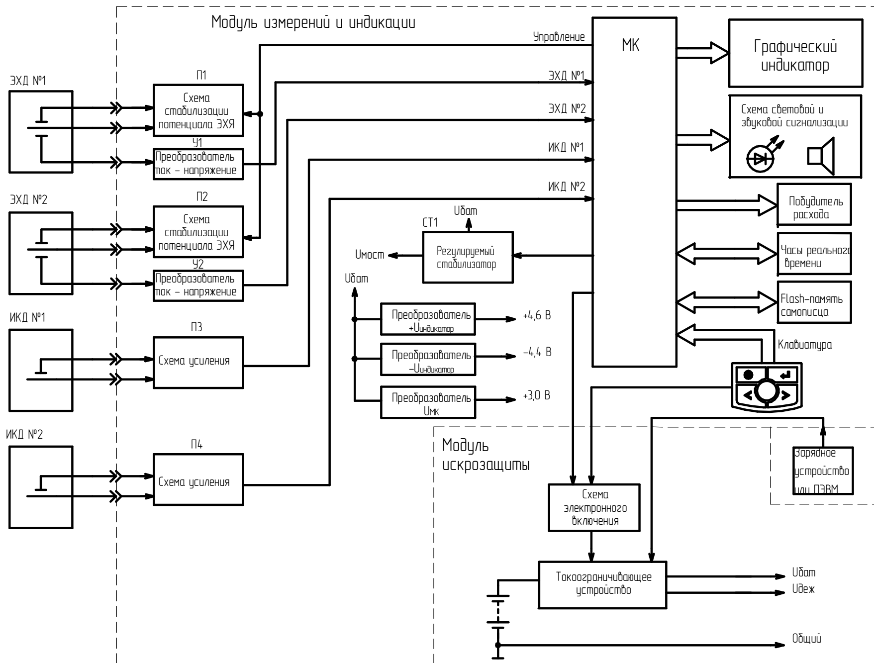
Рисунок 1.4 – Газоанализаторы АНКAT-7664Микро-10 ... -16. Схема функциональная
