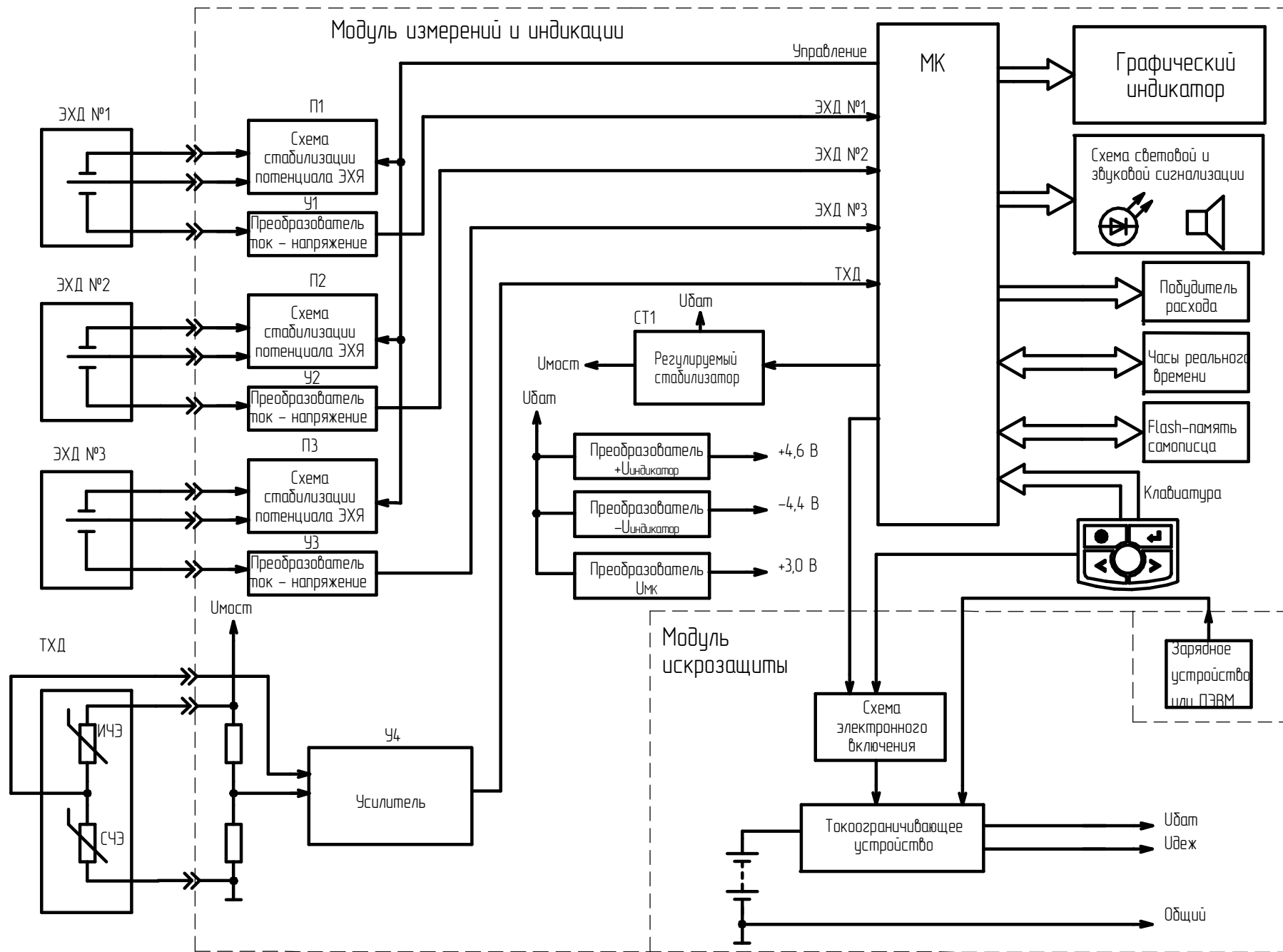
Рисунок 1.2 – Газоанализаторы АНКAT-7664Микро, -01, -03, ... -05. Схема функциональная
