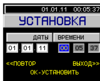
Рисунок 2.10 Установка даты и времени в газоанализаторе
