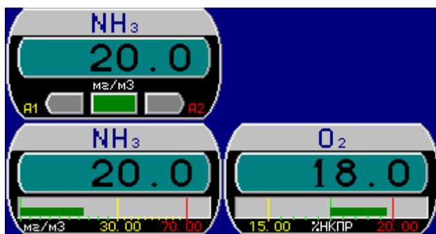
Рисунок 2.4 Вид дисплея газоанализатора в рабочем режиме в различных режимах отображения
