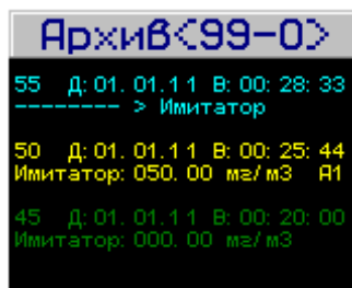
Рисунок 2.9 Пример отображения записи архивных событий
