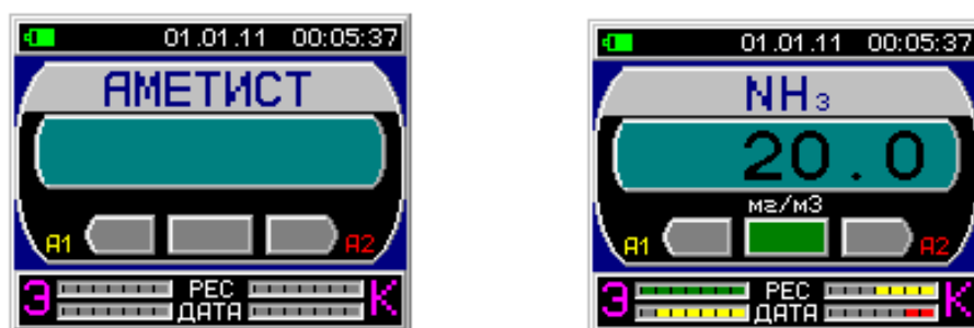
Рисунок 2.1 Вид дисплея газоанализатора в рабочем режиме
