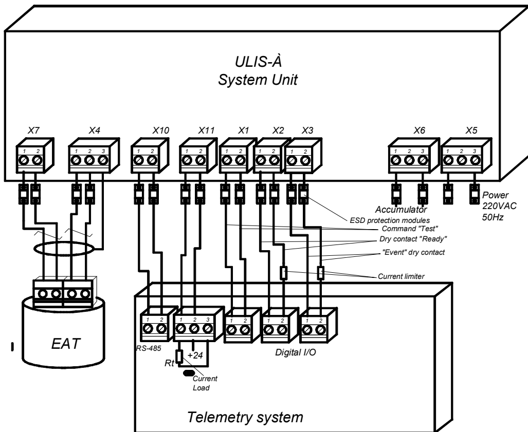
Схема подключения индикатора
