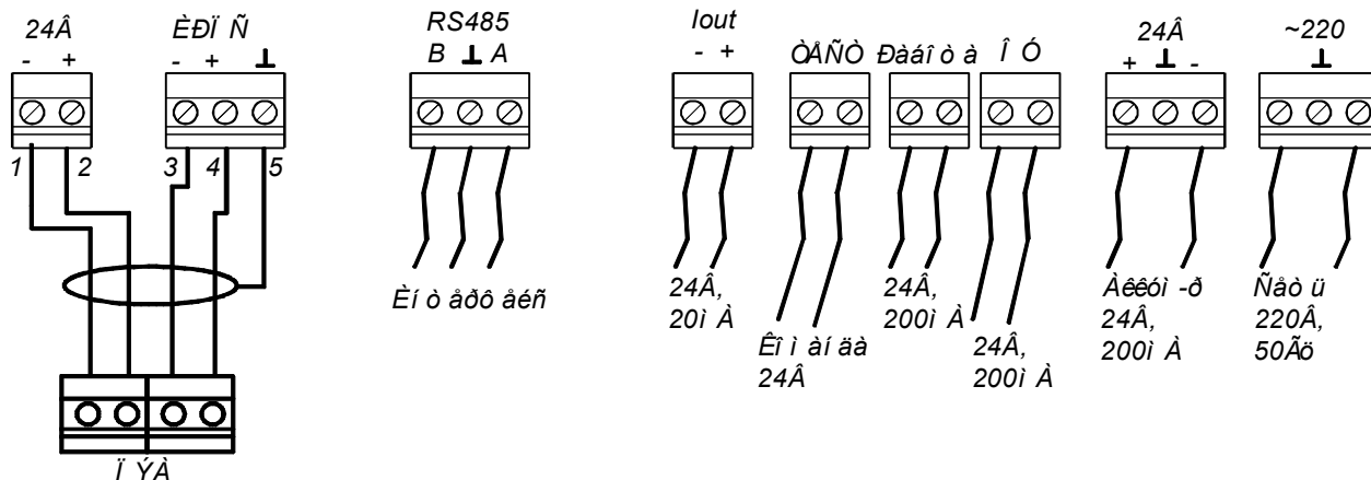
Рис.1. Расположение соединителей
