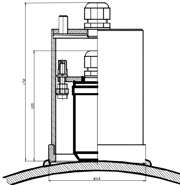
Размещение ПЭА индикатора в монтажном приспособлении
