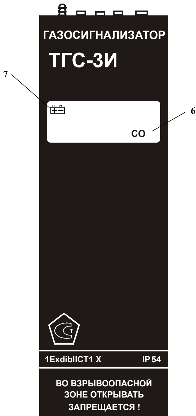
Рисунок 1 Вид передней панели прибора ТГС-3 И
