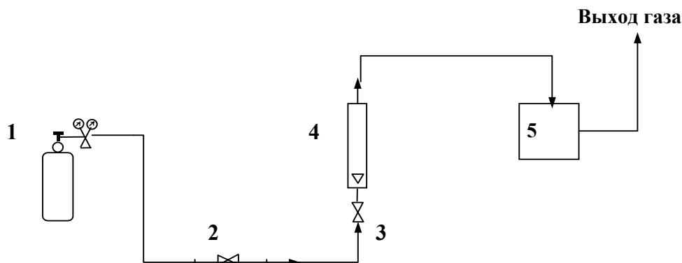
Рисунок 4 Схема подключения прибора ТГС-3 И при поверке.
