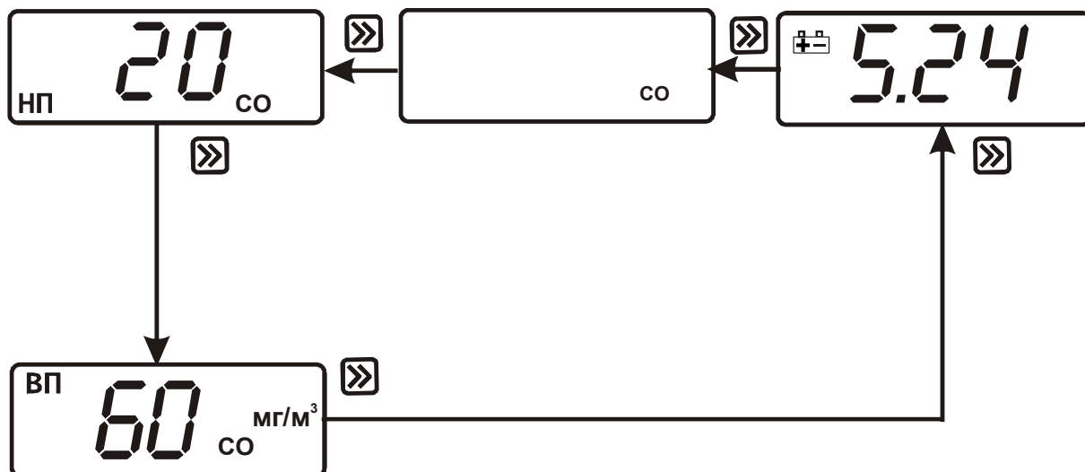
Рисунок 3 Схема вспомогательного режима работы прибора – просмотр порогов
