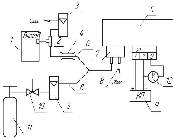
а) для сигнализаторов СТГ-3-Н 2 S, СТГ-3-И-Н 2 S, СТГ-3-SO 2 , СТГ-3-И-SO 2 , СТГ-3-Cl 2 , СТГ-3-И-Cl 2 , СТГ-3-NO 2 , СТГ-3-И-NO 2 и СТГ-3-HCl, СТГ-3-И-HCl (при периодической проверке)
