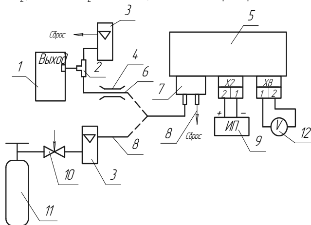
б) для сигнализаторов СТГ-3-Н 2 S, СТГ-3-SO 2 , СТГ-3-Cl 2 , СТГ-3-NO 2 и СТГ-3-HCl (при периодической проверке) с коробкой соединительной
