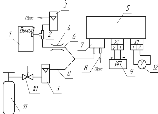
в) для сигнализаторов СТГ-3-И-Н 2 S, СТГ-3-И-SO 2 , СТГ-3-И-Cl 2 , СТГ-3-И-NO 2 и СТГ-3-И-HCl (при периодической проверке) с коробкой соединительной
