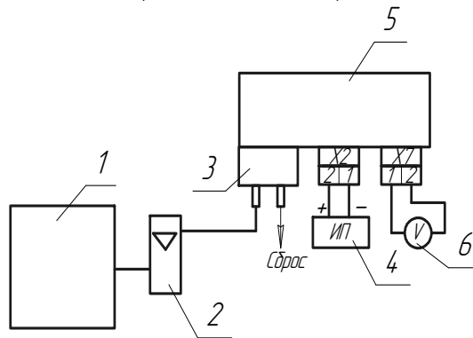
б) для сигнализаторов СТГ-3-НС1 с коробкой соединительной
