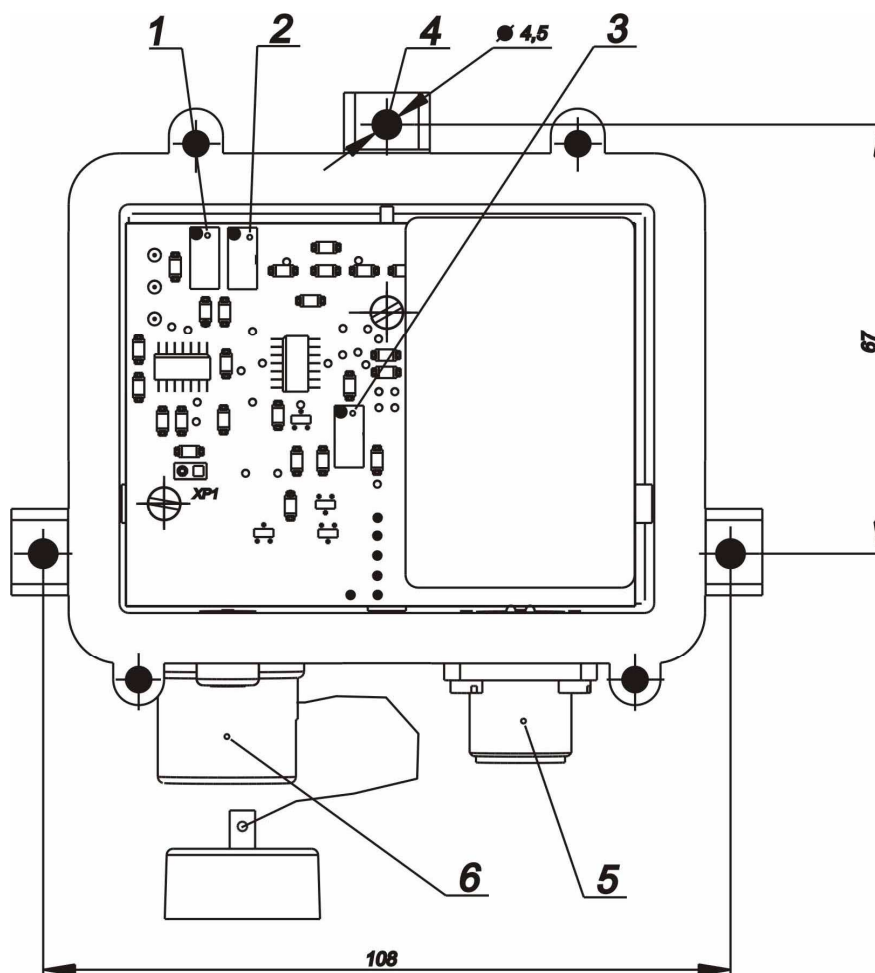
Рис. 2. Датчик в силициновом корпусе со снятой крышкой 1 – потенциометр балансировки моста, 2 – потенциометр регулировки начального тока, 3 – потенциометр регулировки усиления, 4 – установочные отверстия диаметром 4,5 мм, 5 – разъём, 6 – сенсор
