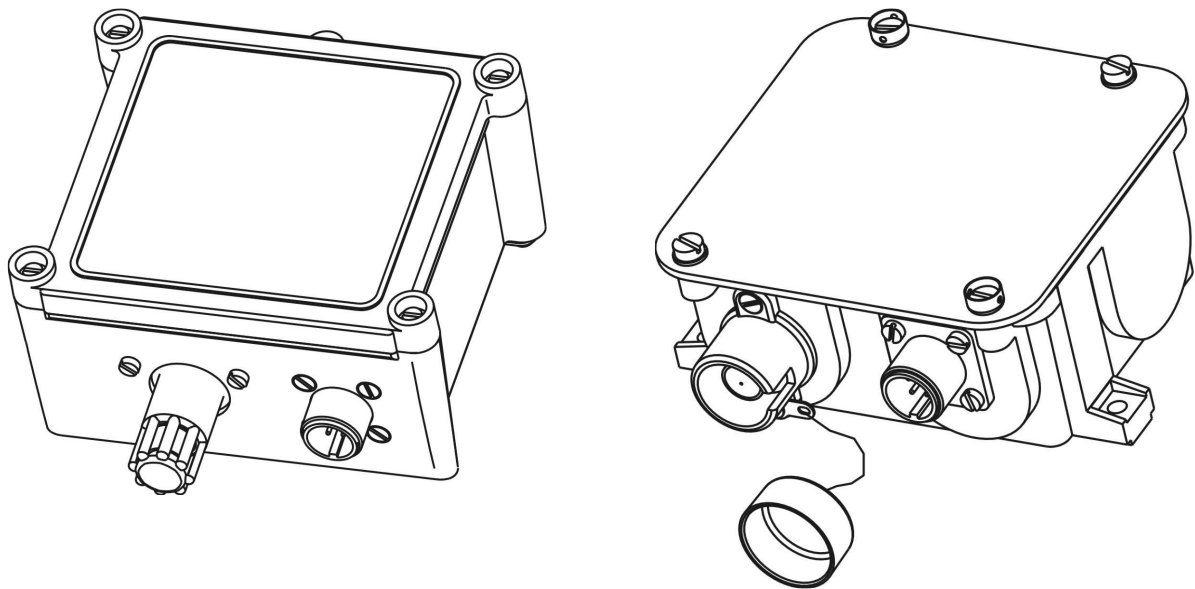
Рис. 1. Внешний вид датчиков в пластмассовом и силициновом корпусе
