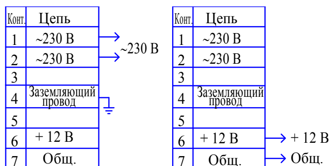
Рисунок 2.1 - Схема подключения газоанализаторов к электрической сети питания
