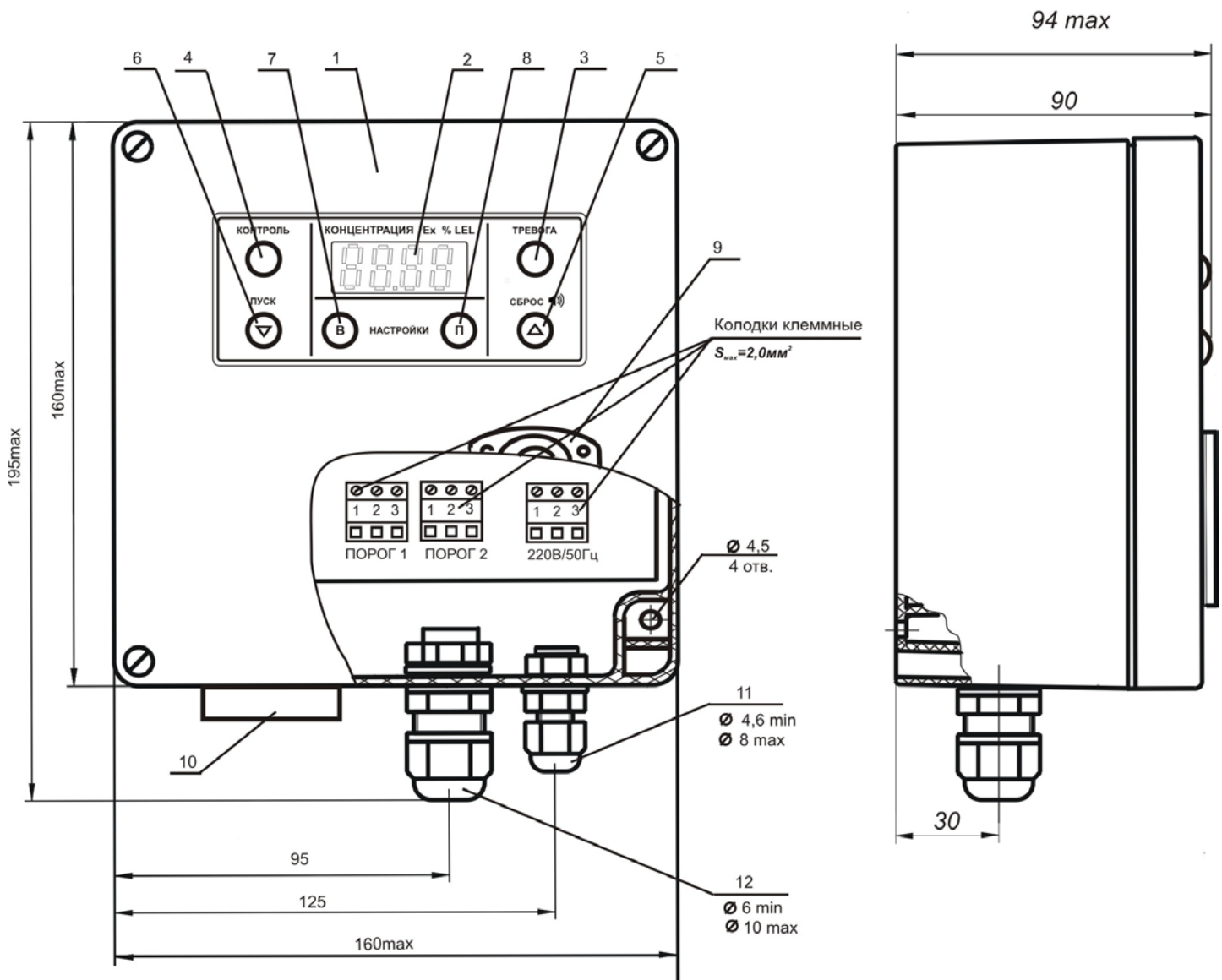
Габаритные, установочные и присоединительные размеры газоанализатора
