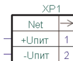
Рисунок 2. Назначение контактов разъема
