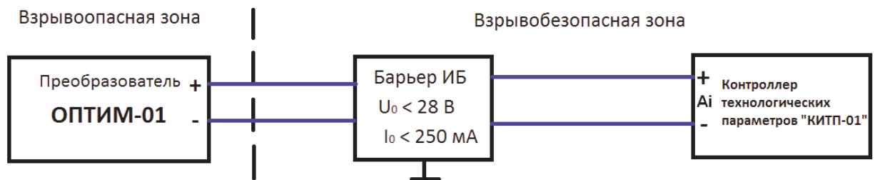
Рисунок А.2 – Схема подключения преобразователя “ОПТИМ-01” контроллеру технологических параметров «КИТП-01».
