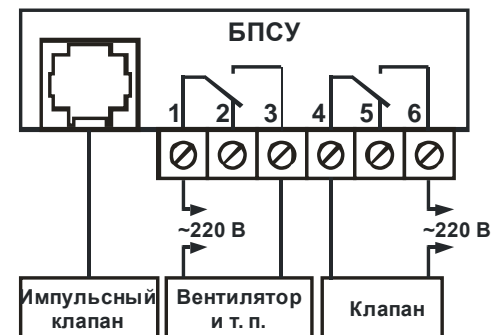
Рисунок 2 – Схема подключения внешнего оборудования к БПСУ
