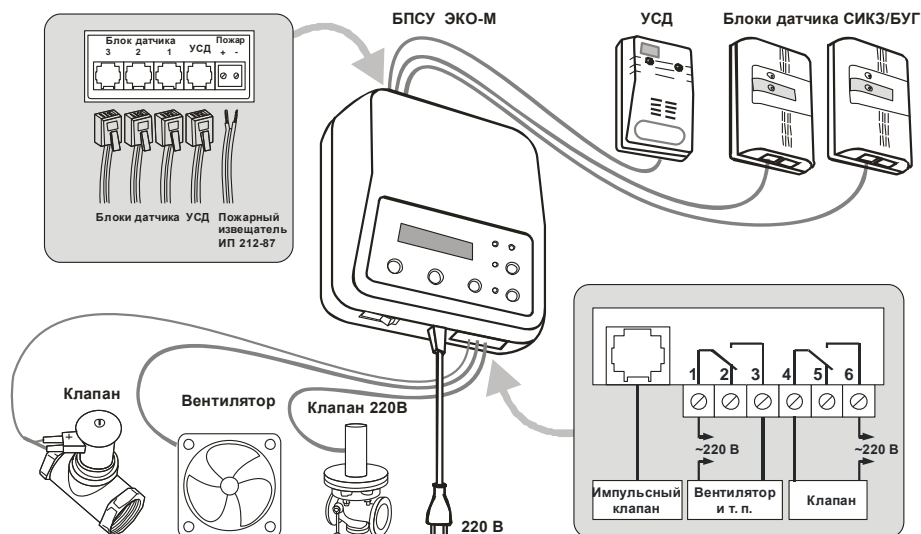
Рисунок 1 – Внешний вид Системы
