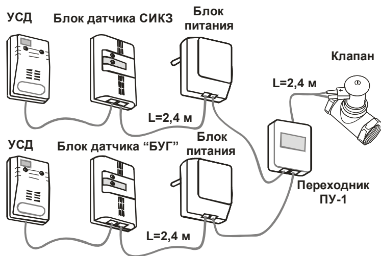
Рисунок 3 – Схема соединения двух сигнализаторов с клапаном
