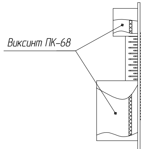
Устройство искробезопасного барьера ИБЯЛ.4.11613.036
